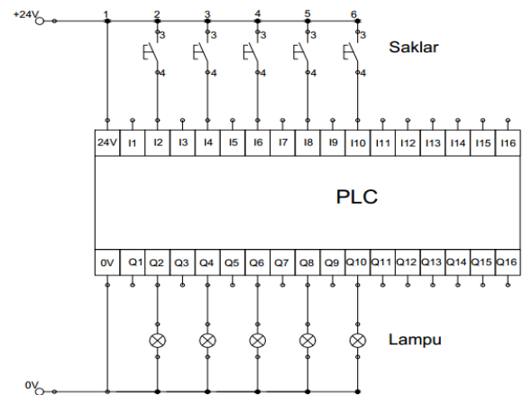
Gambar 5. Pengawatan Pada Perangkat Keras PLC Lantai 1
