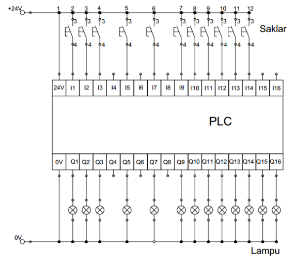
Gambar 6. Pengawatan Pada Perangkat Keras PLC Pada Lantai 2
